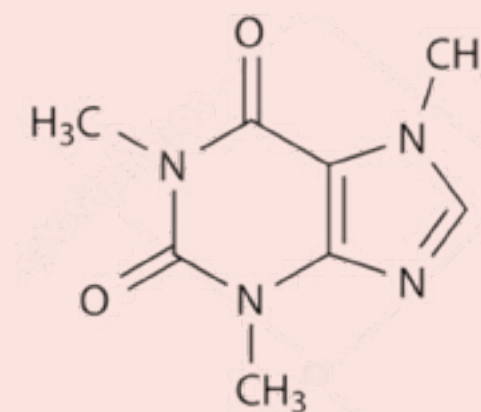
Caffeine
