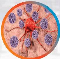
Pomalidomide IH
