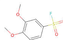
3,4-Dimethoxybenzenesulfonyl fluoride
