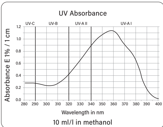
Butyl Methoxydibenzoylmethane
