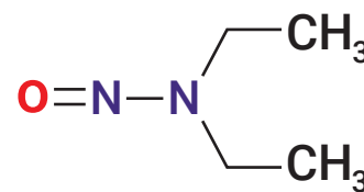
N-Nitrosodiethylamine (NDEA)
