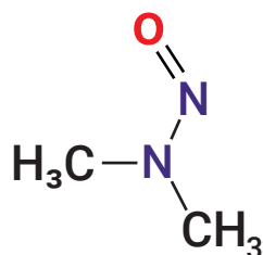
N-Nitrosodiethylamine (NDMA)
